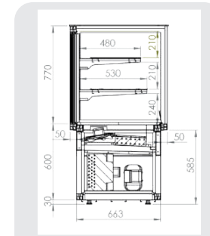
l Detayları Dimension Details
