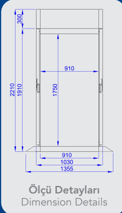
Ölçü Detayları Dimension Details
