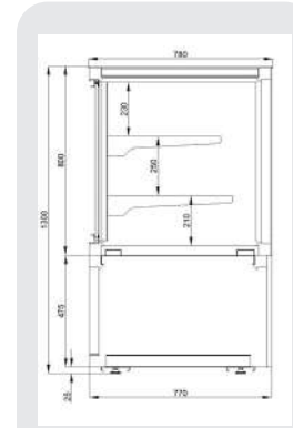
Ölçü Detayları Dimension Details
