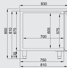
Ölçü Detayları Dimension Details
