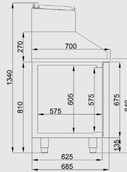
Ölçü Detayları Dimension Details
