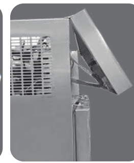
Açılabilir Kanopiyle Kolay Müdahale Olanağı Front Cover Can be Opened For Easy Access
