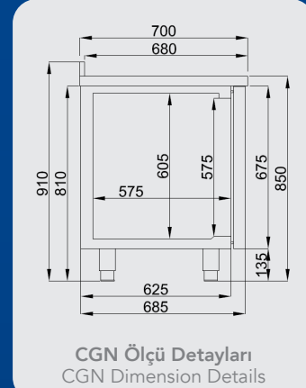
CSN Ölçü Detayları CSN Dimension Details
